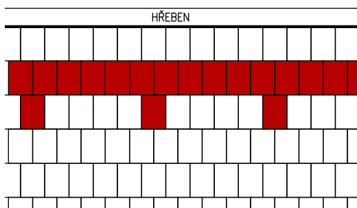
Příklad pro střešní plochu: 18,9 x 8,6 m (74 větracích tvarovek)
