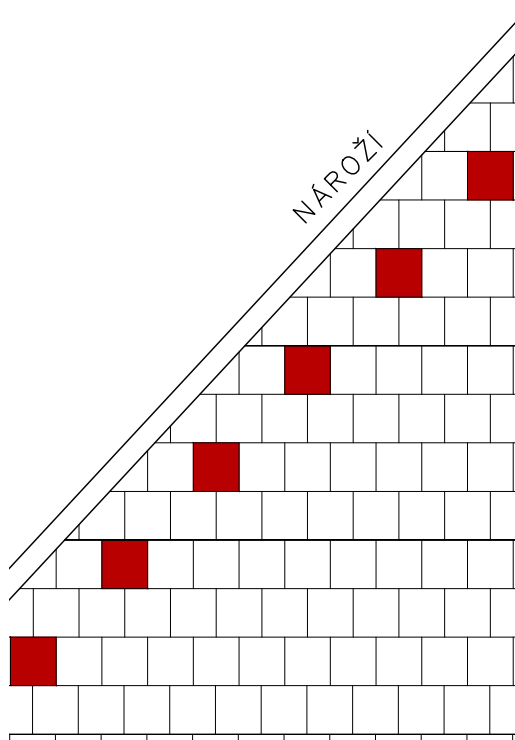
Příklad rozložení v nároží valbové střechy
