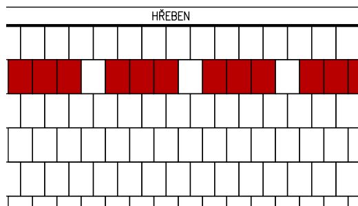
Příklad pro střešní plochu: 11,7 x 5,7 m (30 větracích tvarovek)
